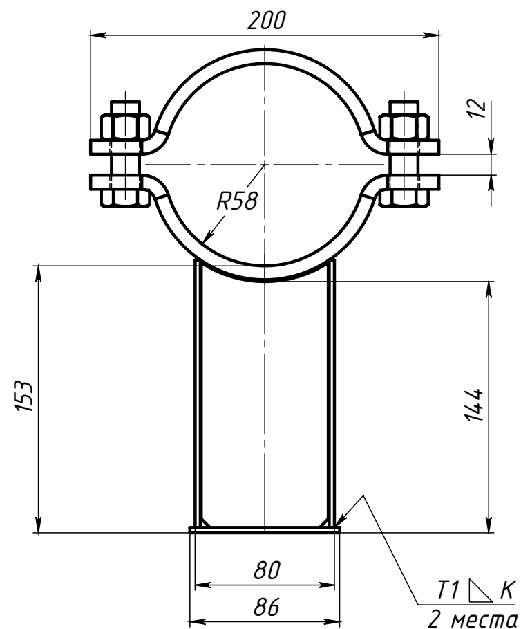
Поз.4 (Полухомут)
